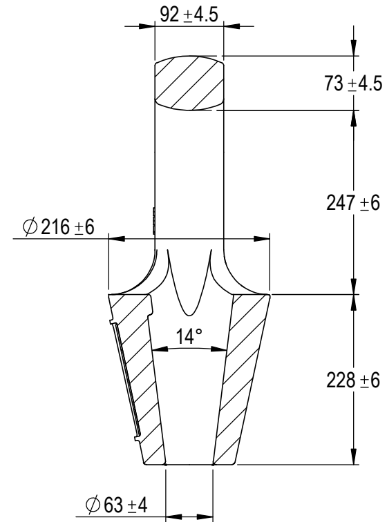
SECTION A-A
