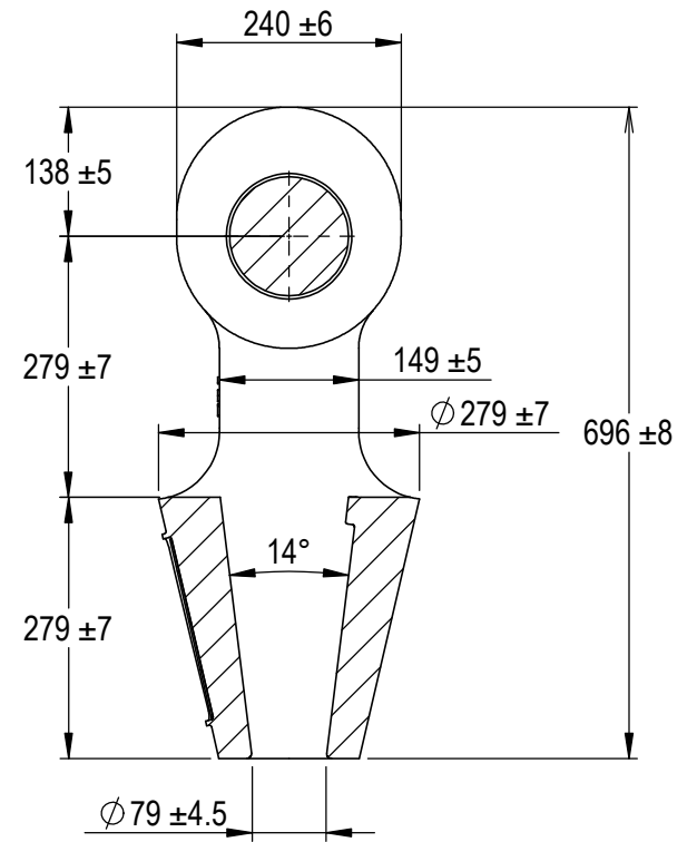
SECTION A-A
